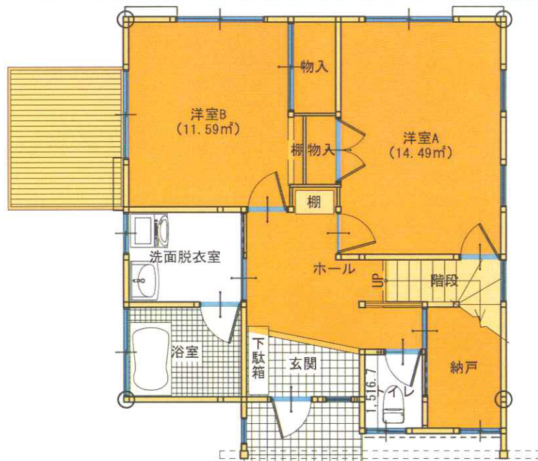
1階 平面図
